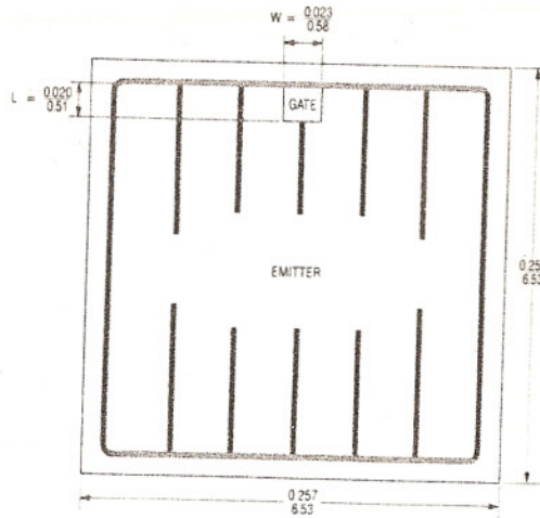
IGBT: HEX-5: 600V
